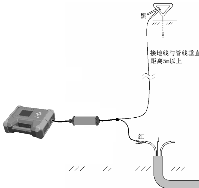
图 7-1-3 接地故障定点接线
