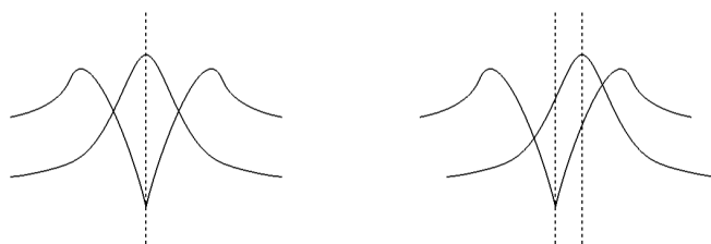
a. 峰谷重合，测深可信
