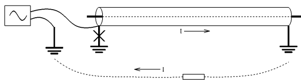
图 3-1-2 护层—大地接线法
