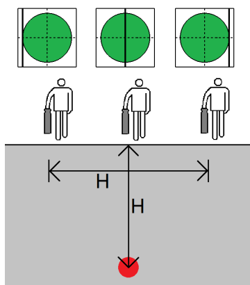
图 5-2-1 罗盘靶标测深
