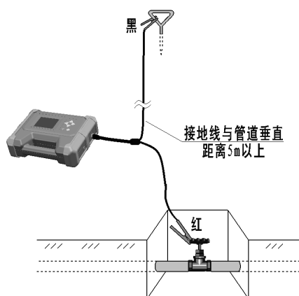
图 2-1-2 直连法接线
