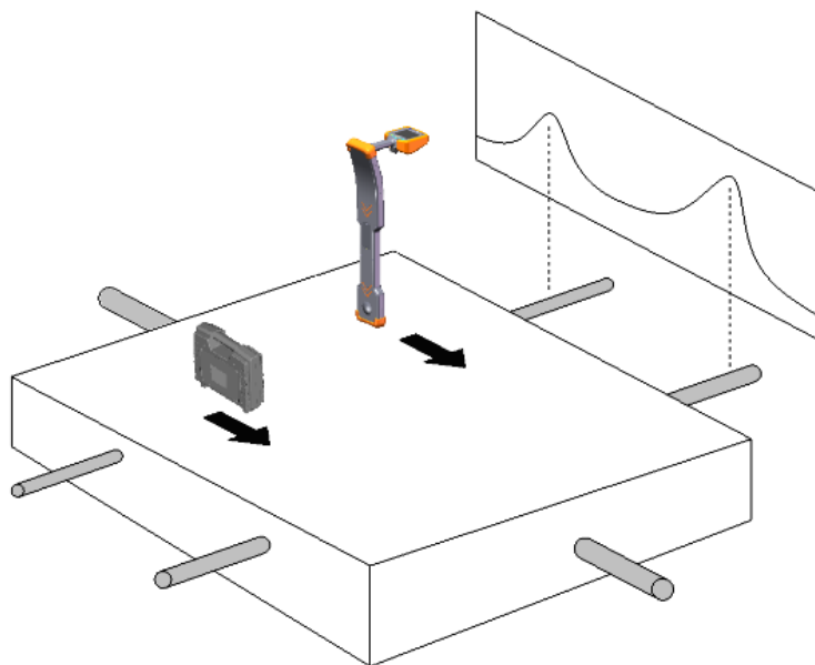
图 4-1-8 辐射法区域探查
