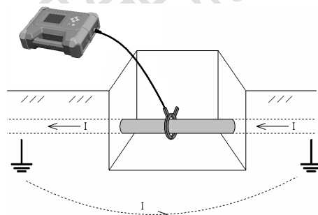
图 2-2-2 卡钳耦合法
