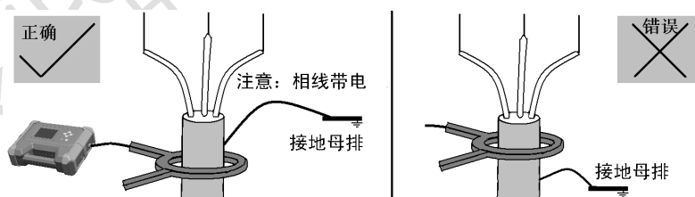
图 3-2-1 运行电缆卡钳耦合法 1（卡电缆本体）
