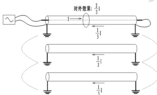
图 3-1-4 并行电缆的分流效果
