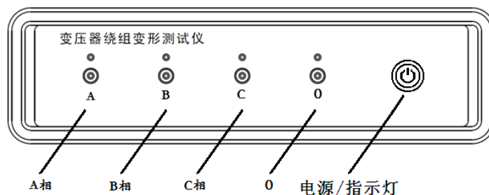
图 1a 变压器绕组变形测试仪面板图(前面板)
