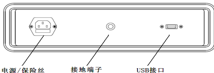
图 1b 变压器绕组变形测试仪面板图(后面板)
