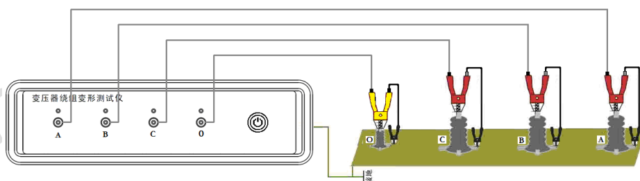
图 2 绕组接线图
