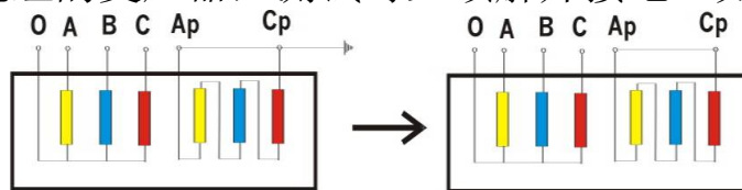
图 3 平衡绕组接线
