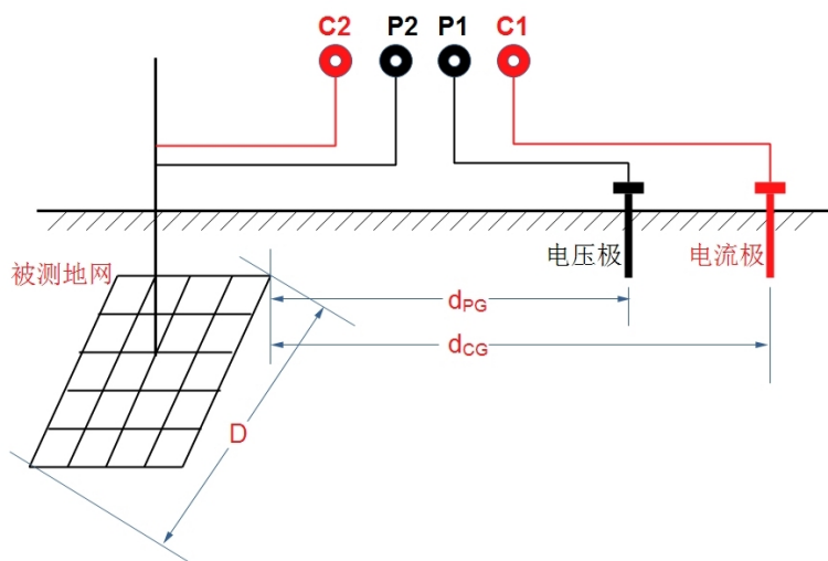
图 5-1 平行布线法测量接线示意图
